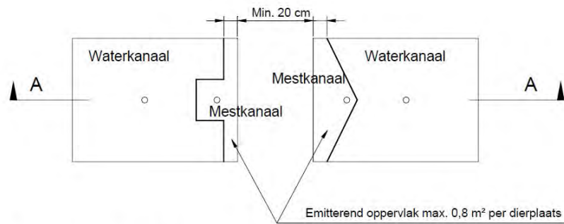
Bovenaanzicht mestpan
