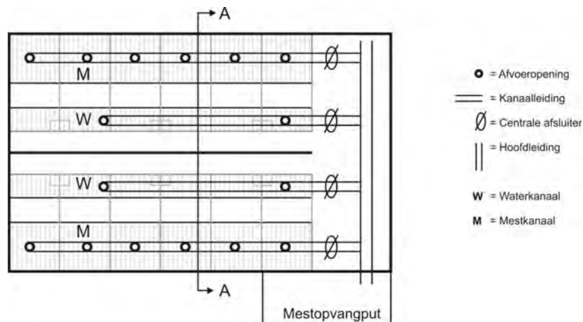
Figuur 47: Doorsnede van een rioleringsysteem. (Bron technisch informatiedocument schuine wanden in stallen voor varkens)
