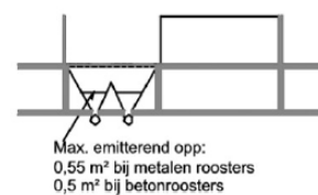
Doorsnede BB
