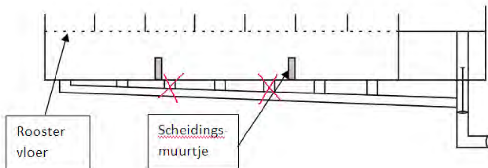
Figuur 48: Mestkelder met scheidingsmuurtjes.
