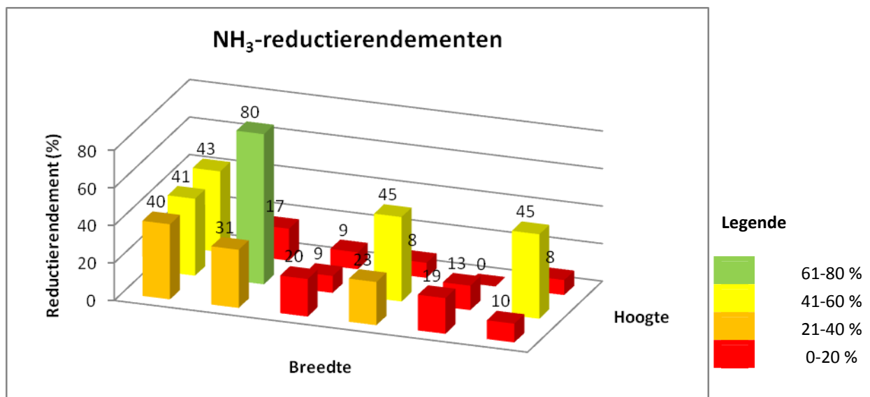
Figuur 19: NH 3 -reductierendementen (%) op de verschillende meetpunten.
