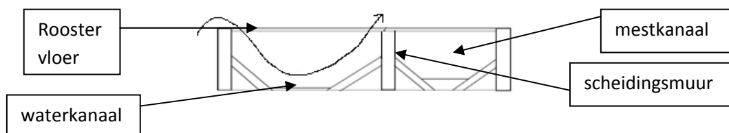
Figuur 23: Ventilatiepatroon bij te brede waterkanalen.
