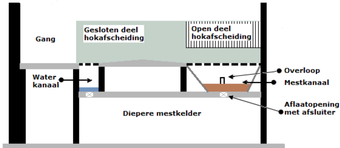
Figuur 1 Schematisch voorbeeld met water- en mestkanaal, dat laatste met twee schuine wanden, en afvoer naar een diepere kelder
