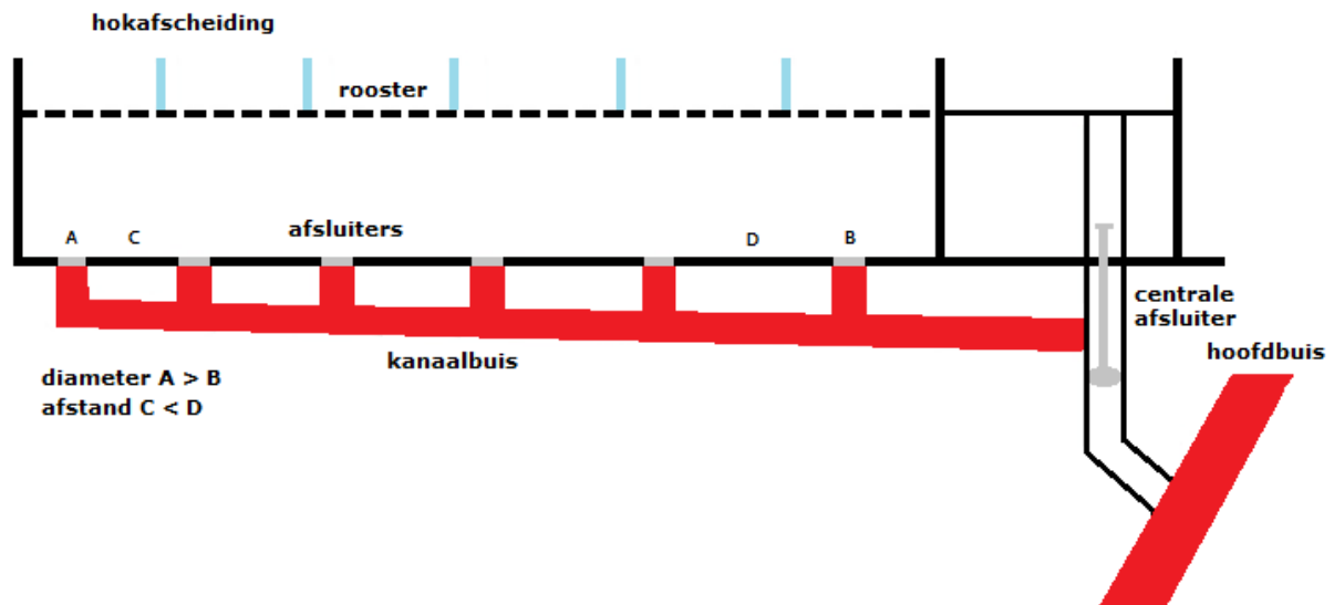
Figuur 2 Schematisch voorbeeld van een rioleringsysteem
