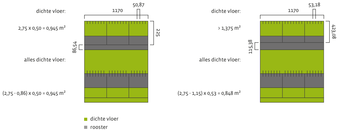
Figuur 4. stalhelft na renovatie tot dropvoederstandjes, rechts met iets bredere gangen
