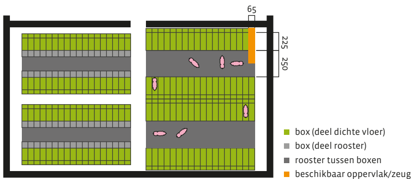
Figuur 2. stal na renovatie tot voederligboxen met uitloop
