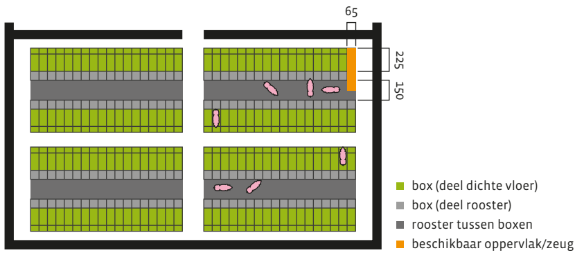
Figuur 1. zeugenstal voor 144 drachtige zeugen, vòòr de renovatie
