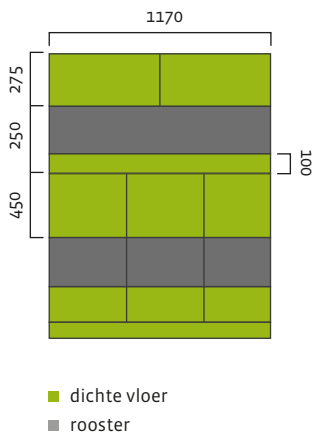
Figuur 5. stal na renovatie tot hokken voor onbeperkte voeding
