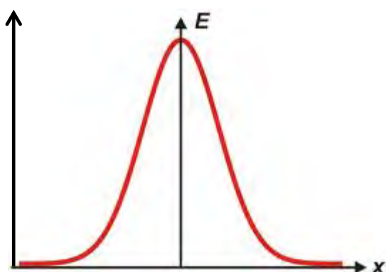
Figuur 12 Normale verdeling met gemiddelde 100 en standaarddeviatie 20
