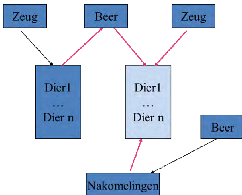
Figuur 10 BLUP- diemodel
