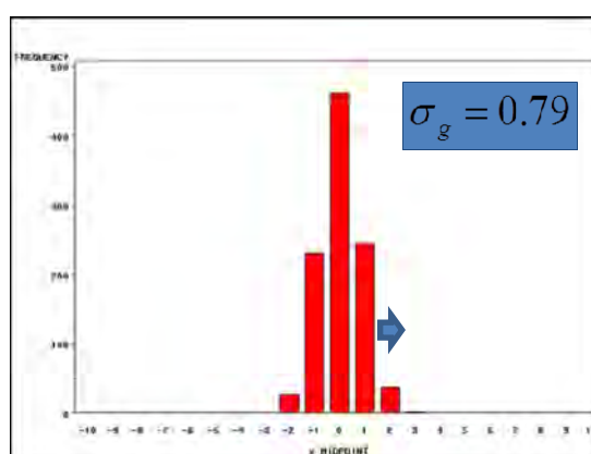
Figuur 9 Spreiding op basis van erfelijke aanleg
