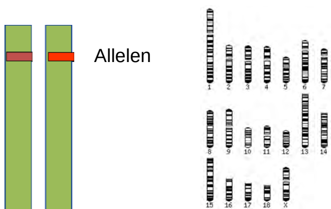
Figuur 18 Schematische voorstelling van chromosomen.
