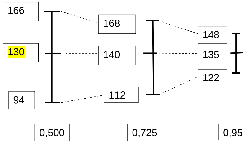
Figuur 11 Betrouwbaarheid van de fokwaardeschatting
