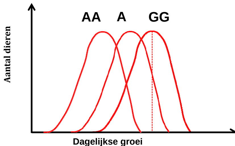
Figuur 21 Verdeling van de dagelijkse groei per genotype
