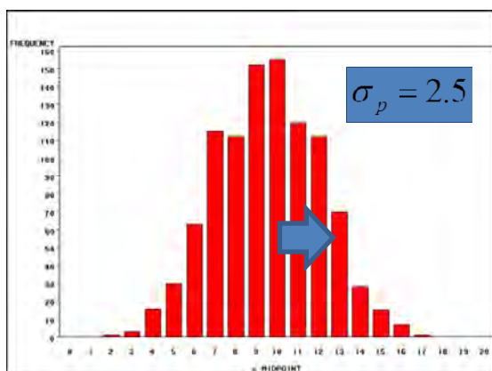
Figuur 8 Waargenomen worpgroottes
