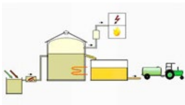
Figuur 13. Biogasinstallatie
